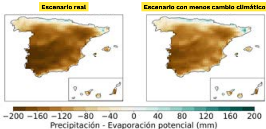
Figura. Mapa de balance hídrico medio mensual (mm mes-1) durante la sequía de primavera 2023 (izquierda) comparado con lo que hubiera sucedido sin el aumento de temperatura de los últimos 30 años (derecha).
