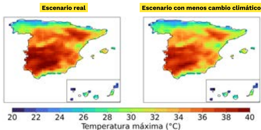
Figura. Mapa promedio de temperatura máxima (OC) durante la ola de calor de 2022 (izquierda) comparado con lo que hubiera sucedido sin el aumento de temperatura de los últimos 30 años (derecha).
